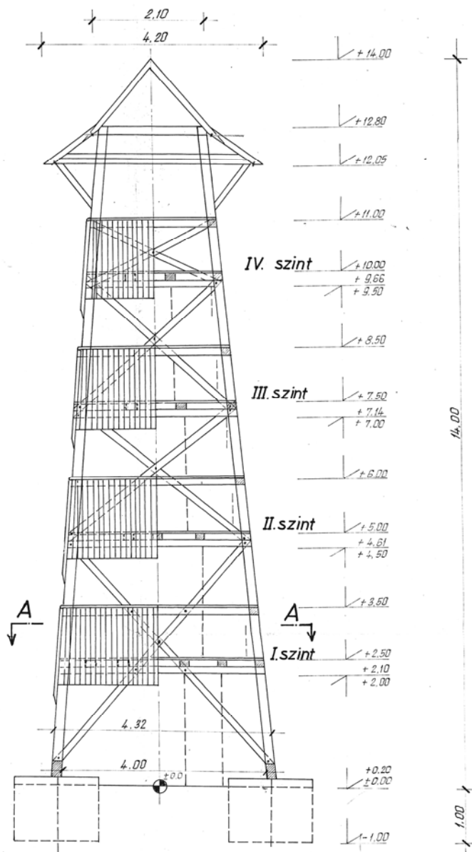
Zalakarosi kilátó homlokzati terve
