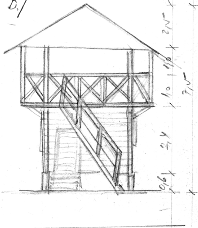
Kiskilátó vázrajz
