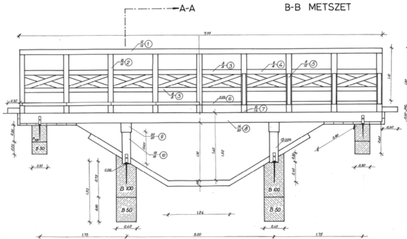
Hosszmetszet
