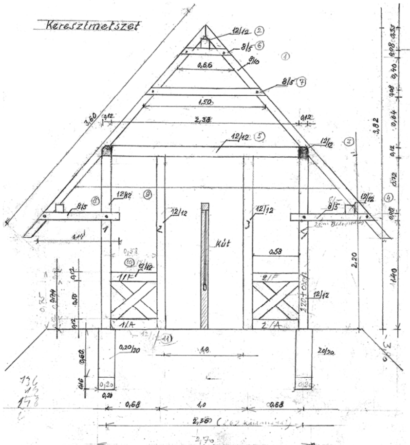
Kútház terv Keresztmetszet
