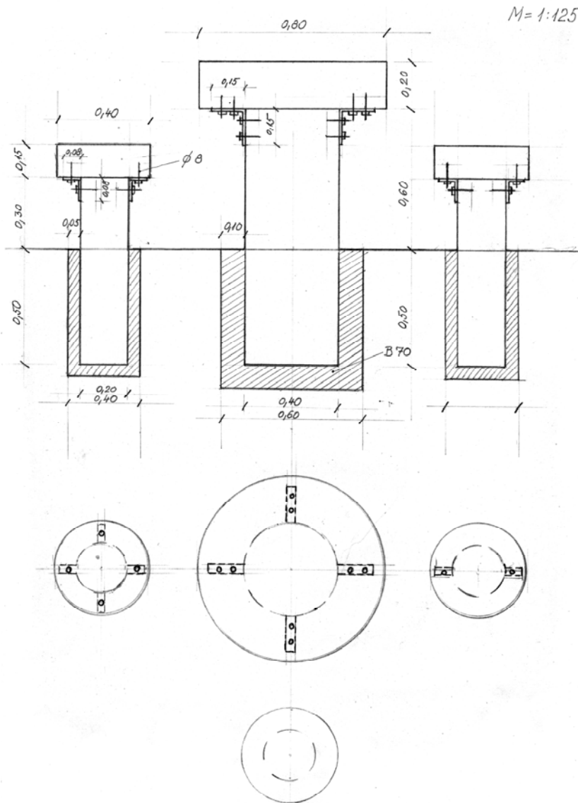
Egy ülőbútorterv a 10 féle közül. Tölgyrönkből fűrészelt, csiszolt, lakozott, betonban.
