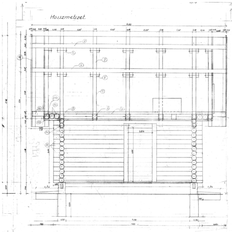
Vendéglátó épület. Hosszmetszet
