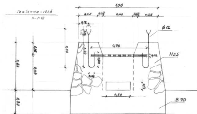
Szalonna-sütő terv betonba ágyazott kövekkel
