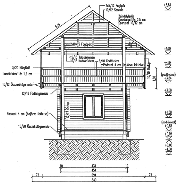
A kilátó és esőbeálló kiviteli terve
