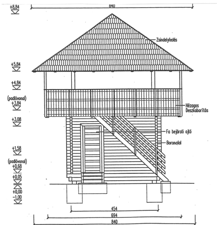
A kilátó és esőbeálló a bejárat és lépcsőfeljáró felől
