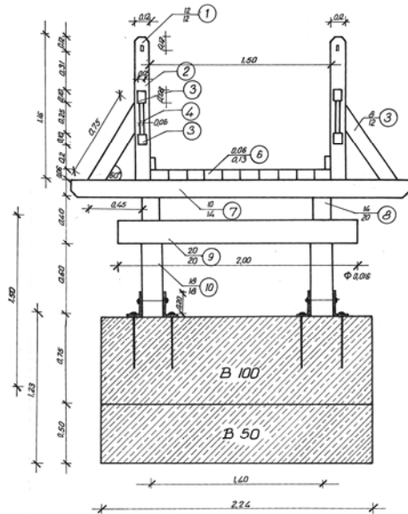
A nagykanizsai parkerdő hidterve. Keresztmetszet
